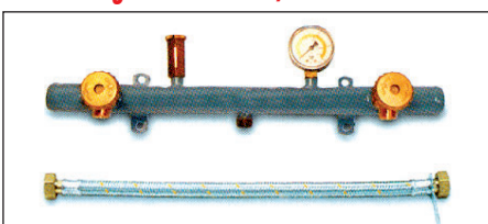
Centralina gas 2 elementi c/manometro e sfiato
